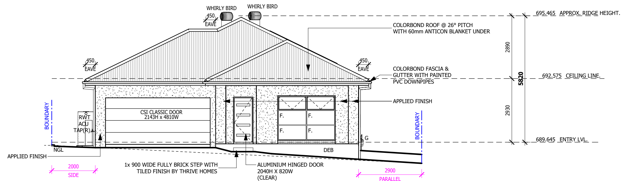
ELEVATION 1
