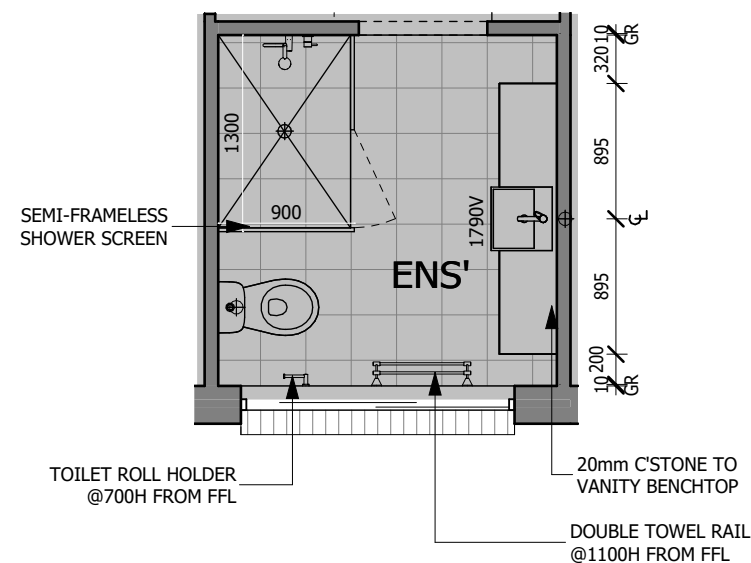
BED 1 ENSUITE
